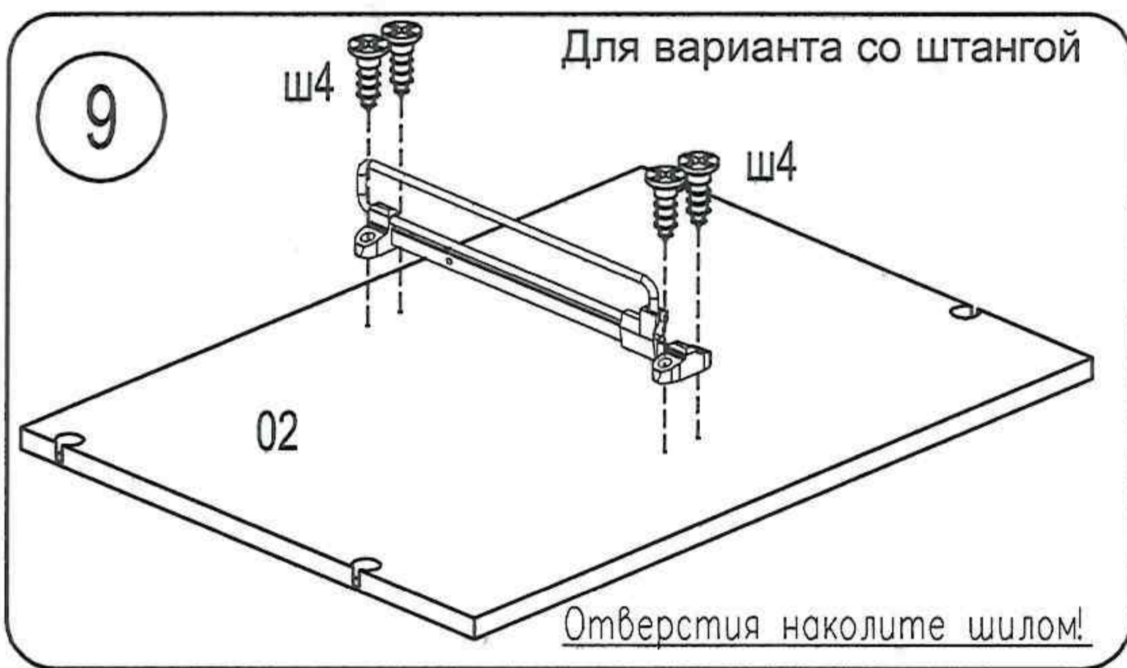
Схема наколок под выдвижную штангу.
