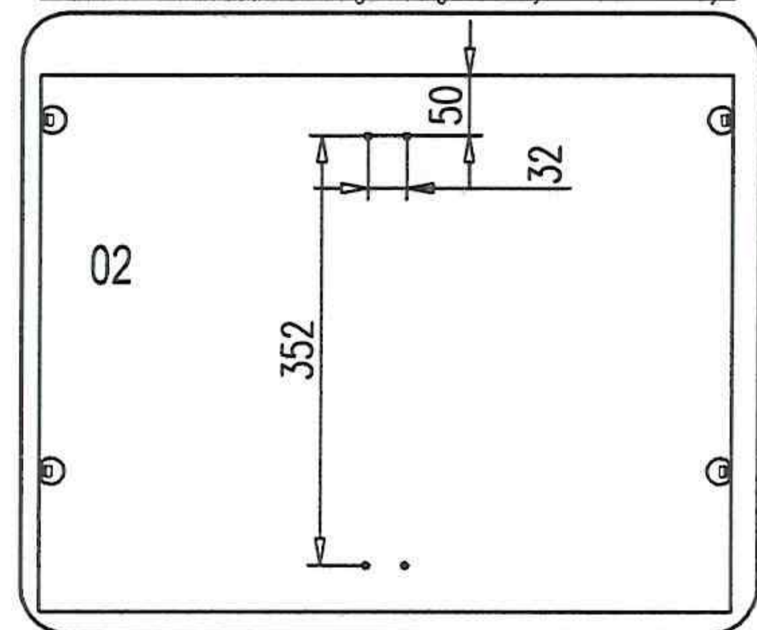
Схема наколок под выдвижную штангу.
